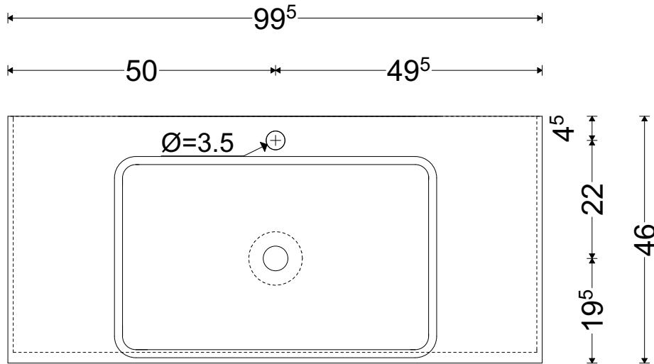
Draufsicht
