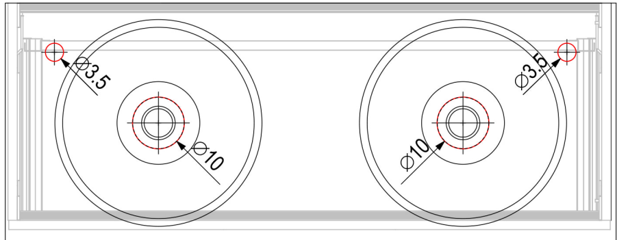
DRAUFSICHT
