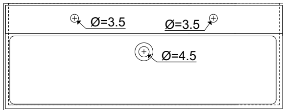
Draufsicht
