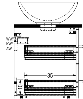
SEITENANSICHT
