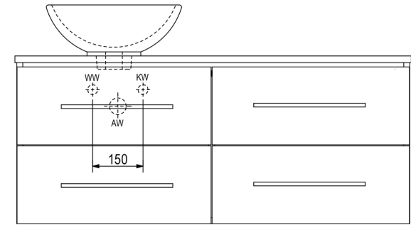
VORDERANSICHT
