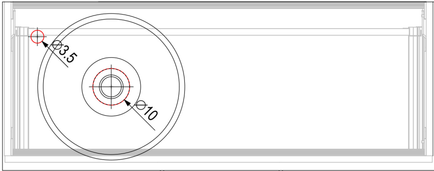
DRAUFSICHT
