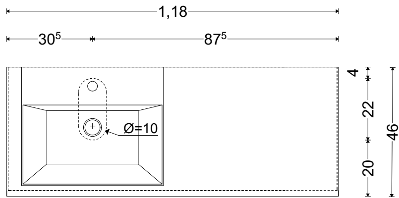
Draufsicht
