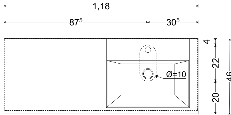
Draufsicht
