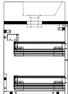
Seitenansicht
